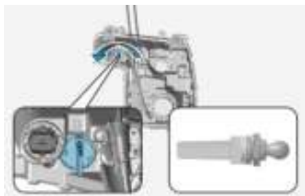
Лампа указателя поворота
